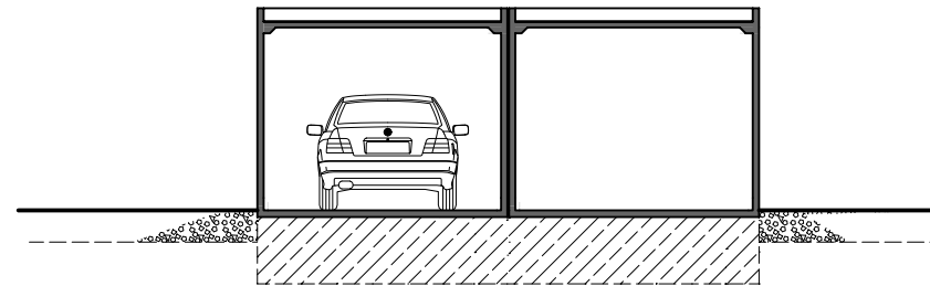
Querschnitt
