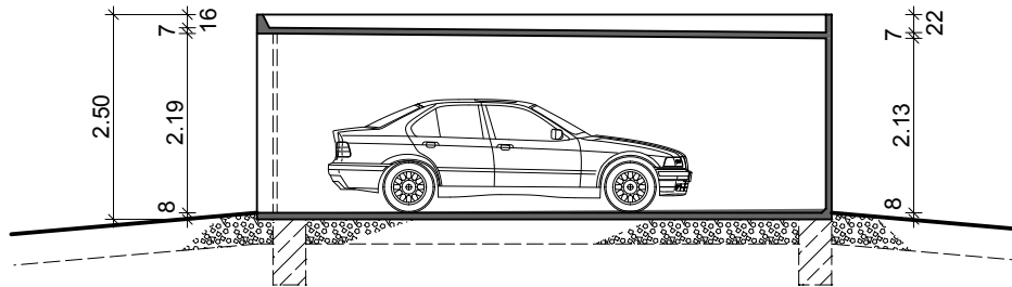
Längsschnitt
