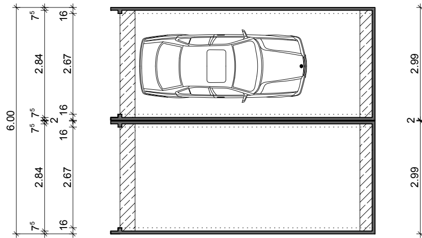
Grundriss
