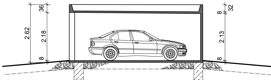
Längsschnitt
