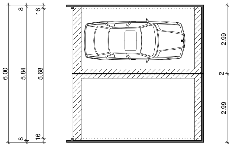
Grundriss
