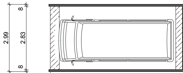
Grundriss
