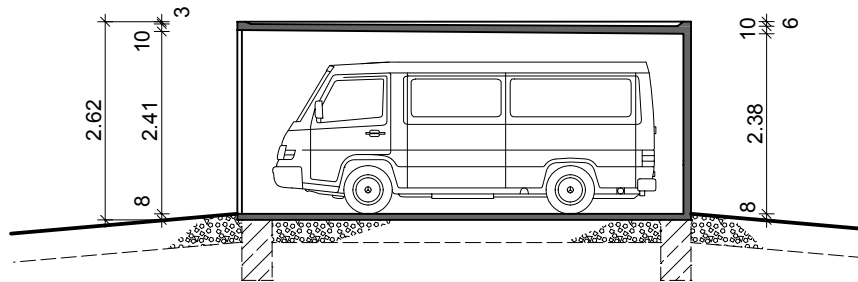
Längsschnitt
