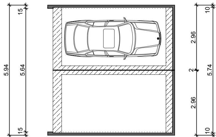
Grundriss
