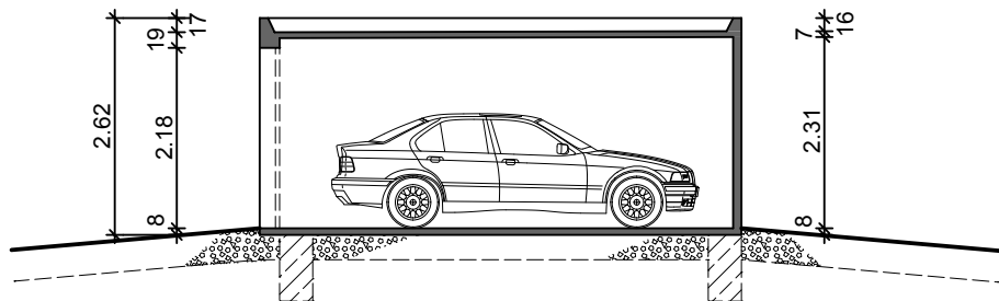
Längsschnitt
