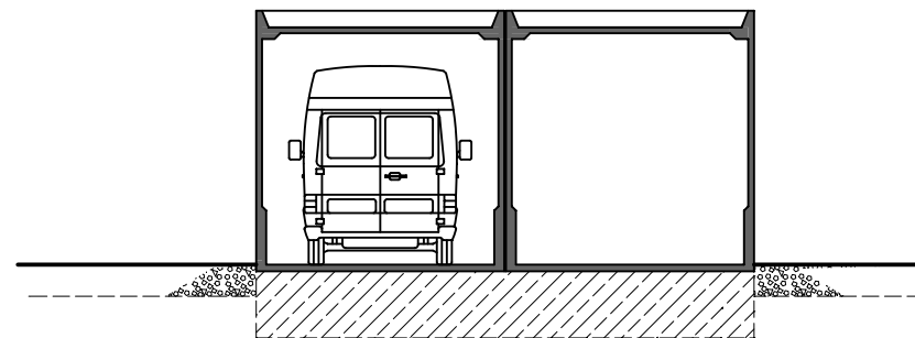
Querschnitt
