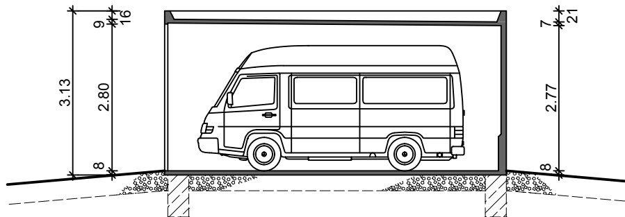
Längsschnitt
