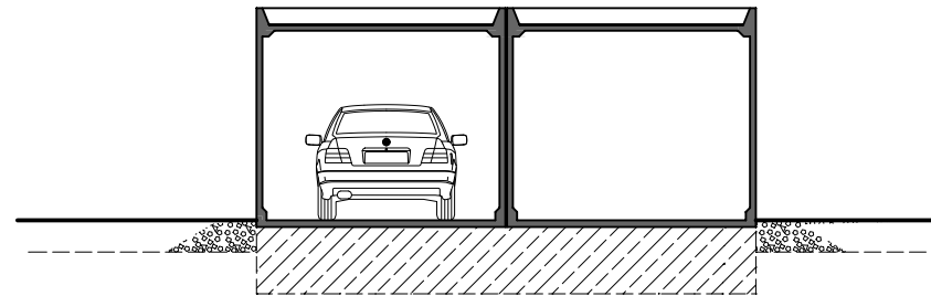
Querschnitt
