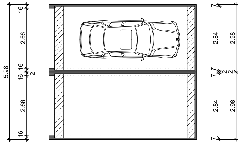
Grundriss
