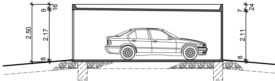
Längsschnitt
