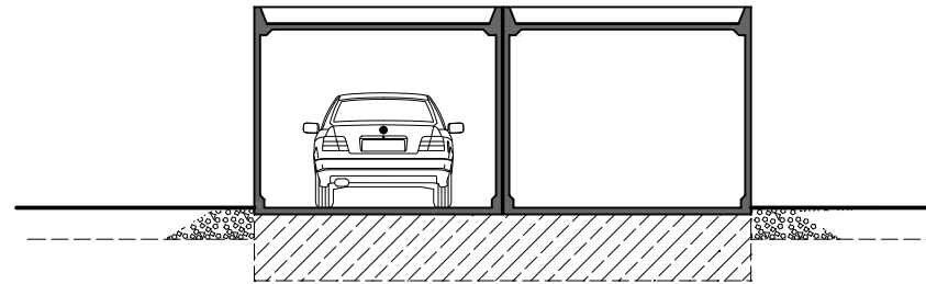
Querschnitt
