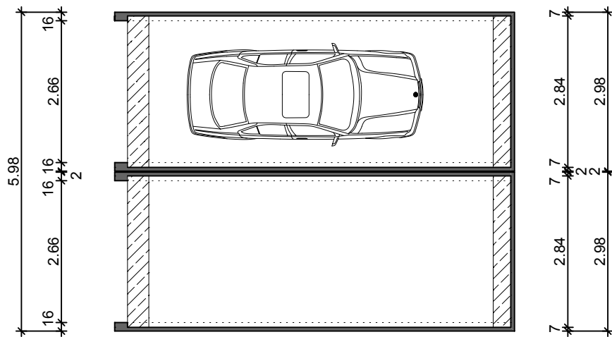
Grundriss
