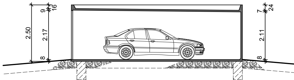
Längsschnitt
