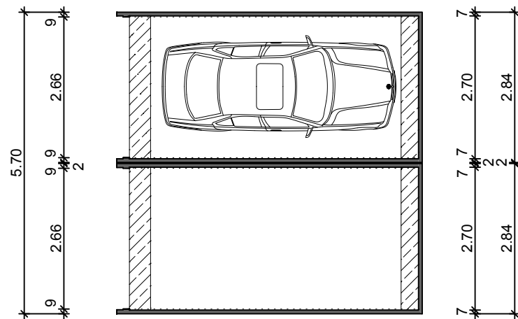
Grundriss
