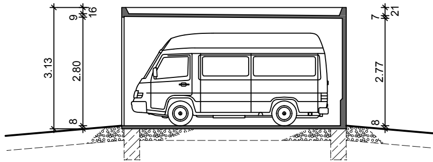
Längsschnitt
