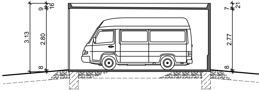
Längsschnitt
