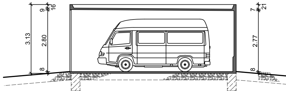
Längsschnitt
