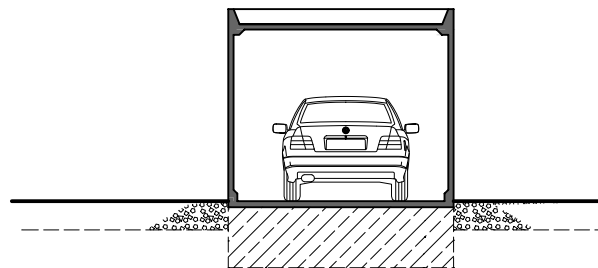
Querschnitt
