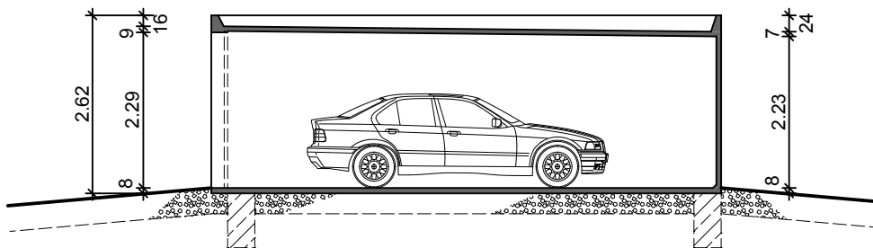
Längsschnitt
