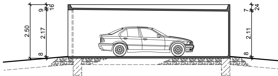
Längsschnitt
