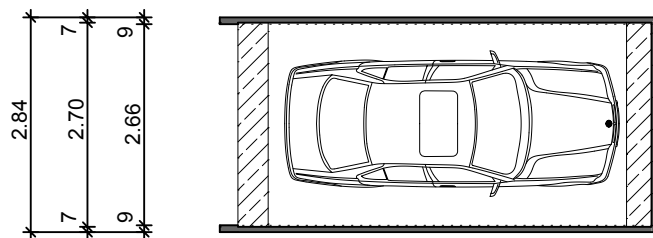
Grundriss
