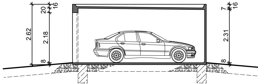
Längsschnitt
